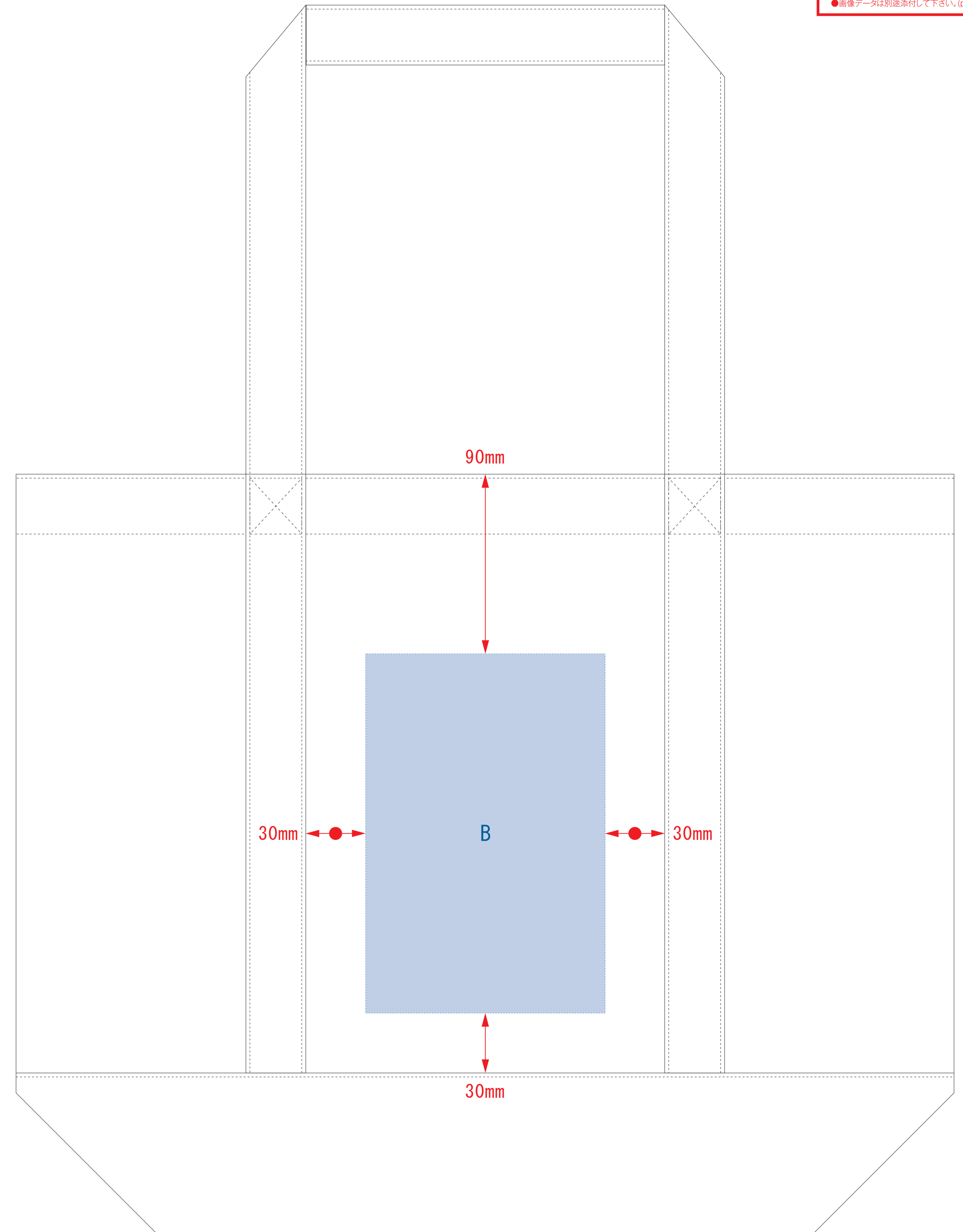
裏面
